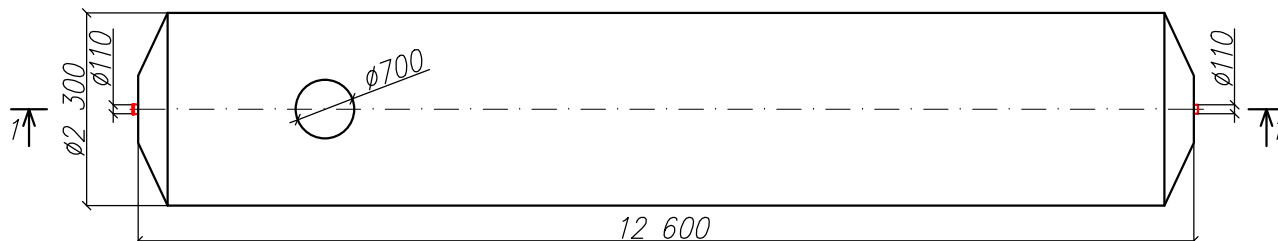
Вид сверху
